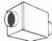
Modèles 3 ou 7 plénum 2 gaines GH 25 : Ø 313 - Ø 313 GH 50 : Ø 313 - Ø 313 GH 80 : Ø 400 - Ø 400 GH 120 : Ø 500 - Ø 460
